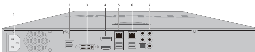
图1-4 TL-VMS600后面板示意图
